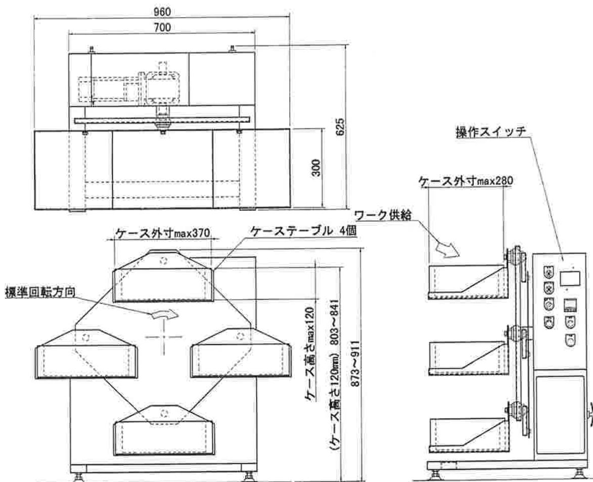
回転ストッカー PSG型 標準寸法
