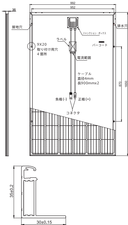
太陽光発電モジュール図面 単位:mm
