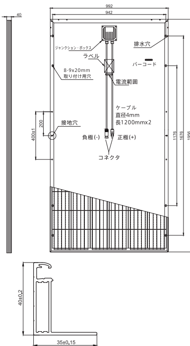
太陽光発電モジュール図面 単位: mm
